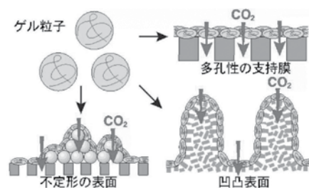
アミン含有ゲル粒子膜の成膜方法の模式図。ゲル粒子水溶液を、さまざまな表面構造を有する多孔性の支持膜表面にスプレー塗工するだけで、欠陥のないガス分離膜を成膜することが可能である。（九大プレスリリース）
