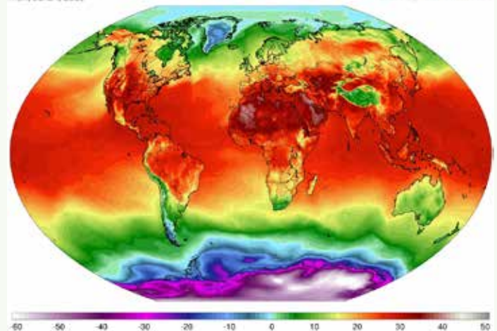
CFSv2 Avg 2m Temperature (°C) Mon, Jul 24, 2023
